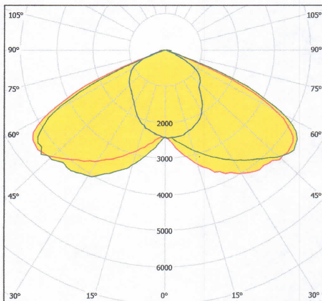
Рисунок 5 – КСС образца светильник светодиодный LED UniLED ECO-MS 50-115W (мощность 75,2 Вт) в поперечной (C0-C180) (красная кривая), продольной (C90-C270) (синяя кривая) плоскостях и плоскости максимальной силы света (C184-C4) (зеленая кривая)
