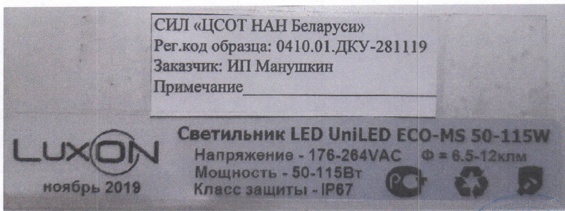
Рисунок 8 – Фотография маркировки и регистрационной этикетки образца светильник светодиодный LED UniLED ECO-MS 50-115W
