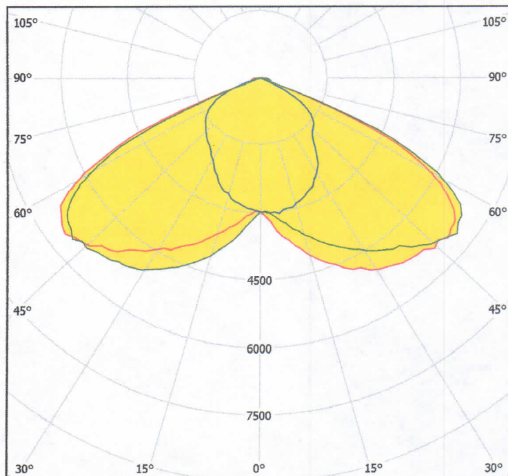
Рисунок 1 – КСС образца светильник светодиодный LED UniLED ECO-MS 50-115W (мощность 121,6 Вт) в поперечной (C0-C180) (красная кривая), продольной (C90-C270) (синяя кривая) плоскостях и плоскости максимальной силы света (C178-C358) (зеленая кривая)
