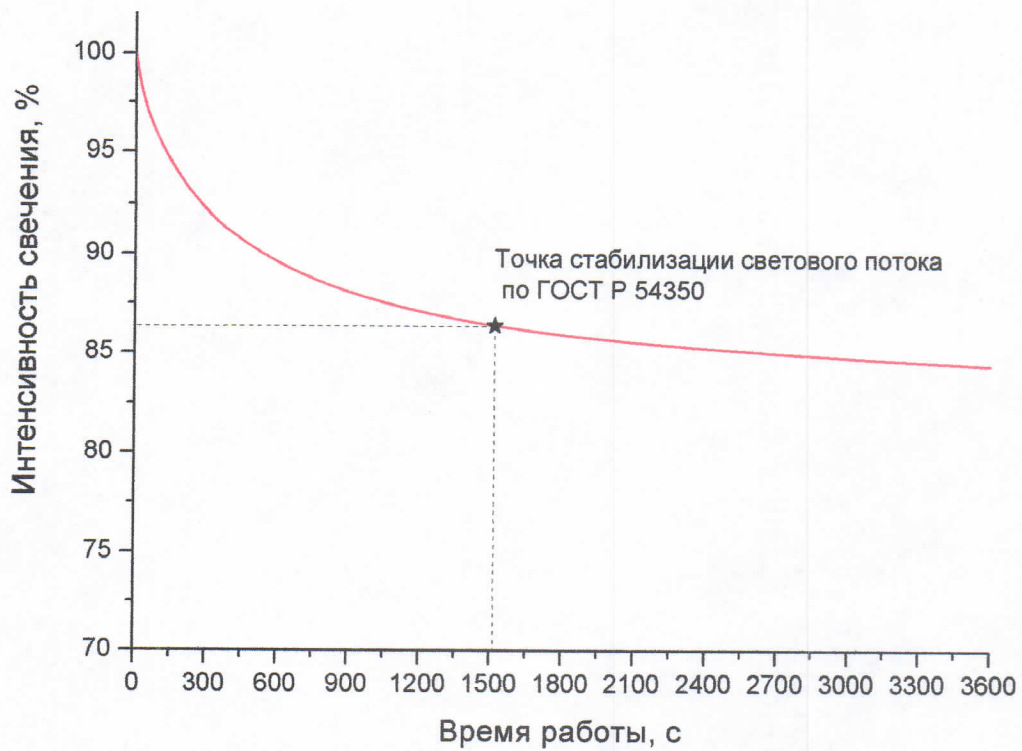
Рисунок 3 – График стабилизации светового потока образца светильник светодиодный LED UniLED ECO-MS 50-115W (мощность 121,6 Вт)
