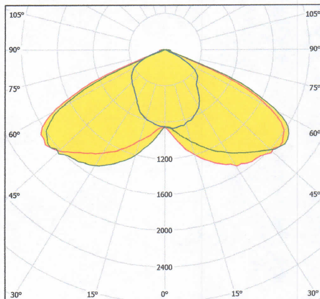
Рисунок 6 – КСС образца светильник светодиодный LED UniLED ECO-MS 50-115W (мощность 24,0 Вт) в поперечной (C0-C180) (красная кривая), продольной (C90-C270) (синяя кривая) плоскостях и плоскости максимальной силы света (C182-C2) (зеленая кривая)
